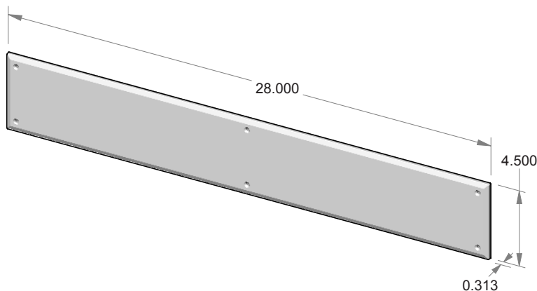
KP-284.5 – Bevel Edge kick plate.
