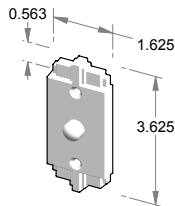
DRB-761 – Deco door bell plate. – Matching solid bronze button.
